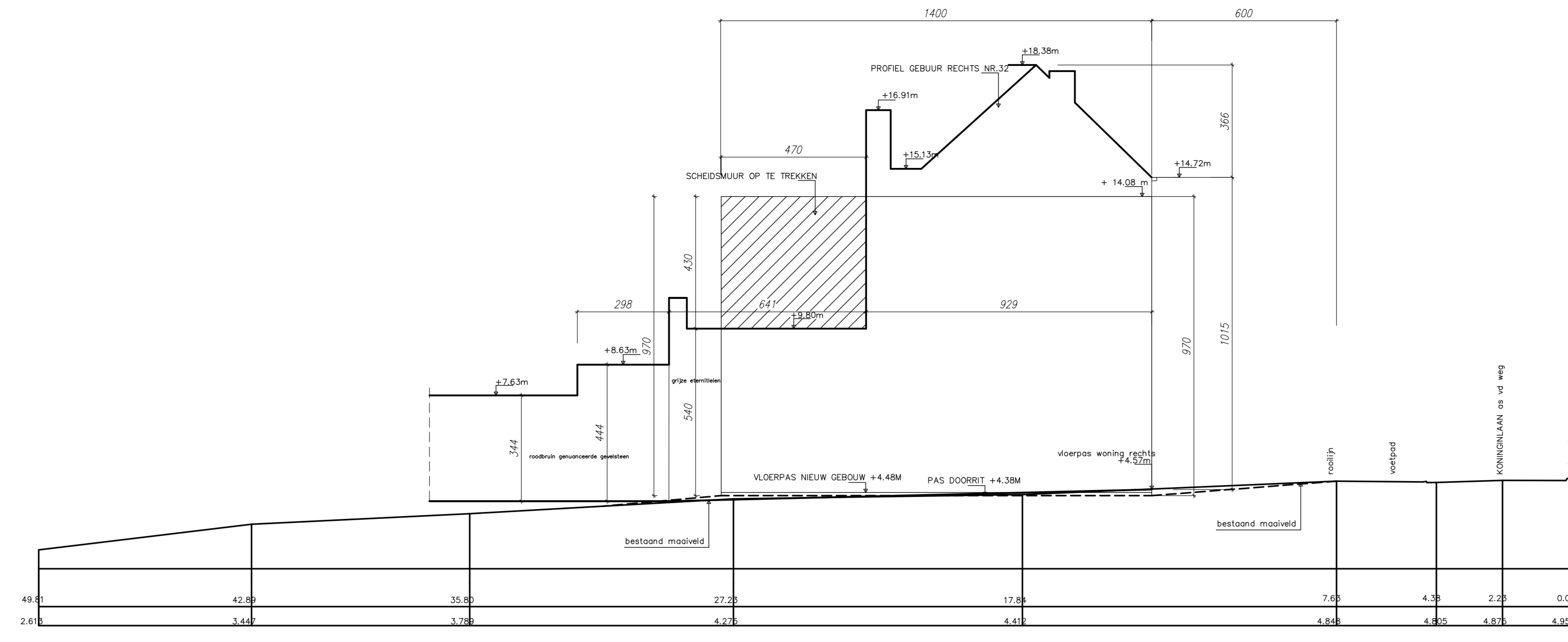
TERREINPROFIEL aa op rechterperceelsgrens schaal 1/100
