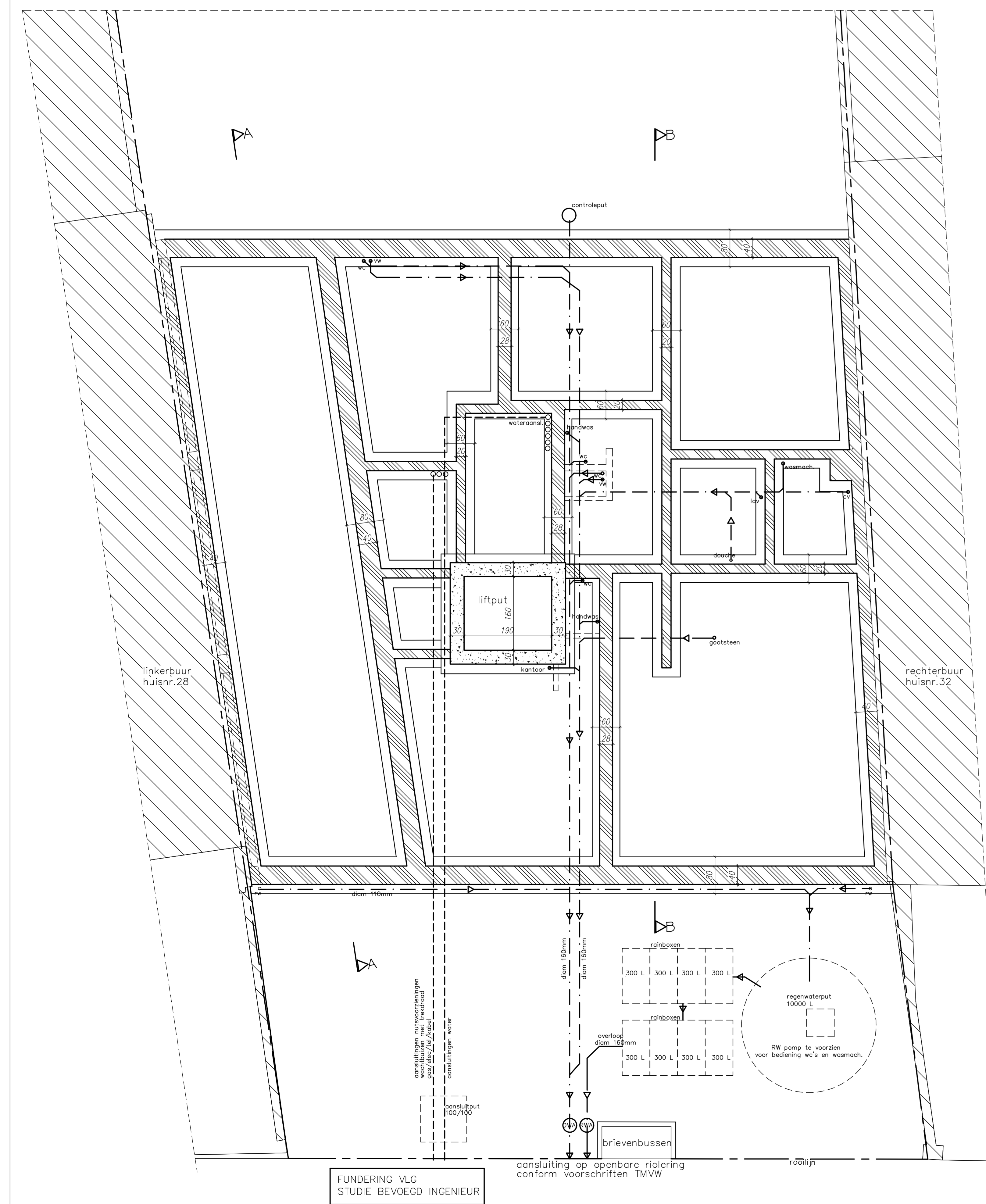
Funderings- en rioleringsplan schaal 1/50
