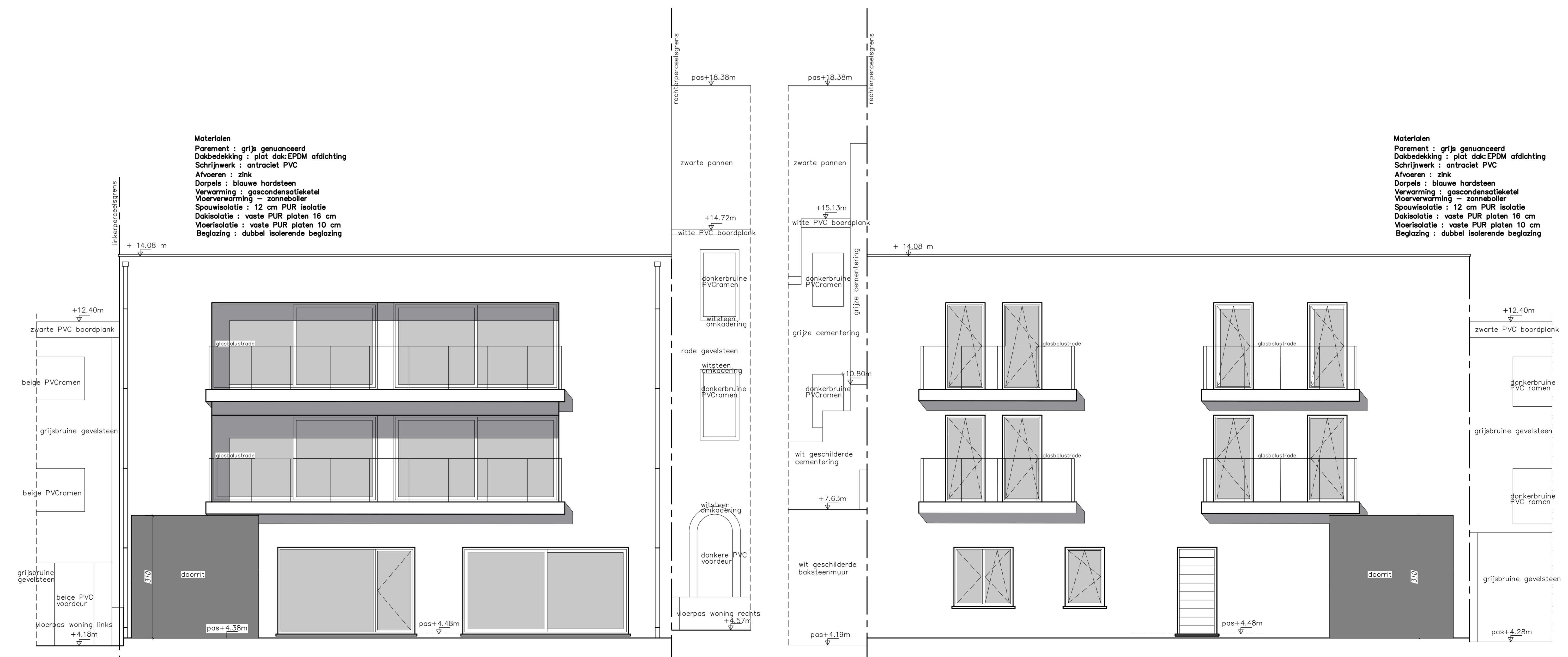
VOORGEVEL schaal 1/50
