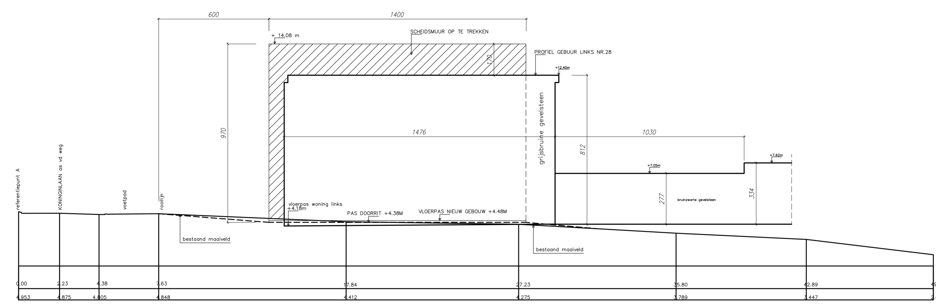
TERREINPROFIEL bb op linkerperceelsgrens schaal 1/100
